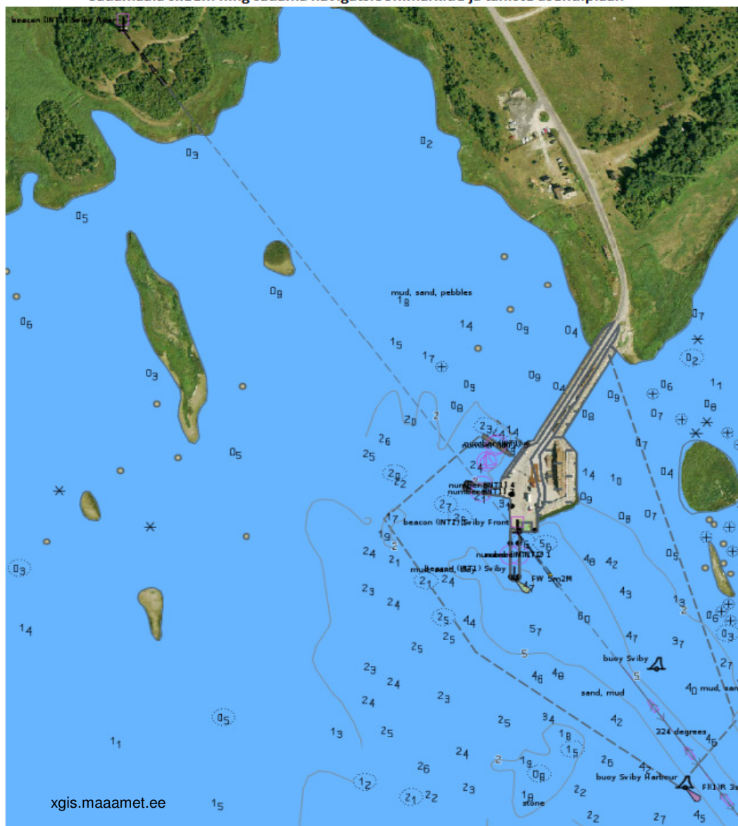
Sadamaala skeem ning sadama navigatsioonimärkide ja tähiste asendiplaan
